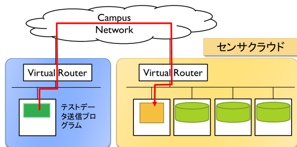
図 4 性能評価実験の環境
