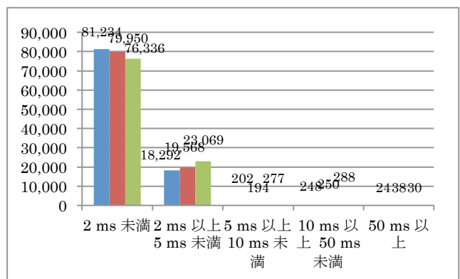
図 6 各試行の処理時間分布
