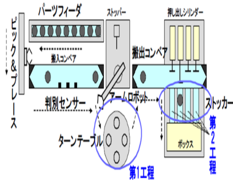
図 6 FA 実験装置
