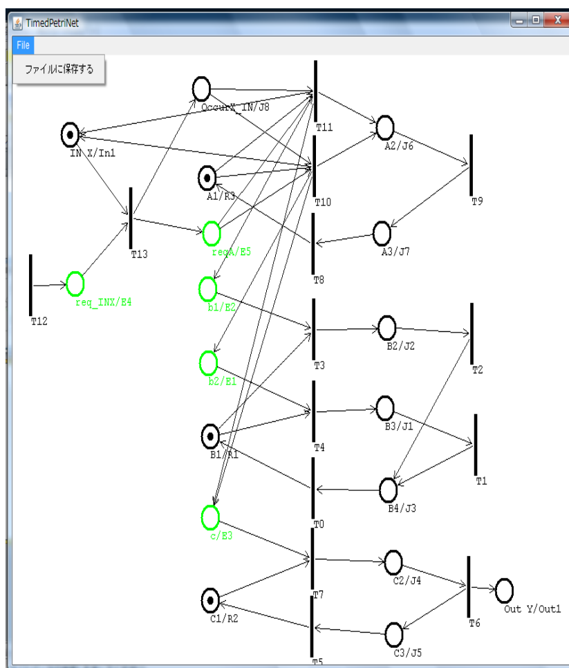
図 5 ETSC を時間ペトリネットへ変換した例
