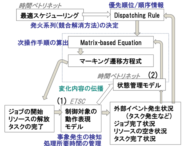
図 2 MDEC2 の枠組み
