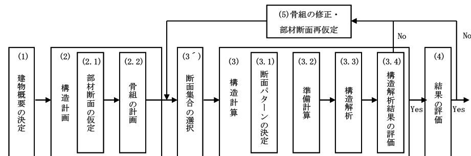
図6 本手法を用いた鋼構造設計の流れ
