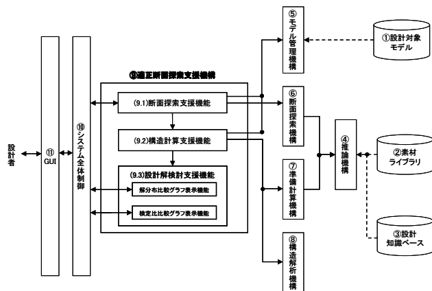
図 9 適正断面探索支援機構の構成
