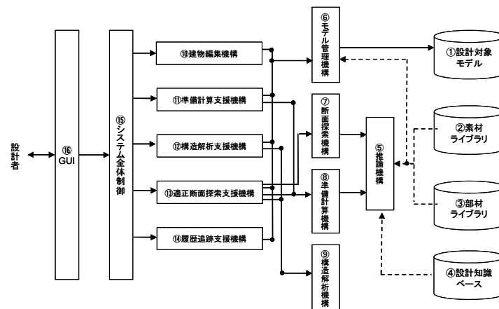
図 8 鋼構造設計教育支援システムの構成
